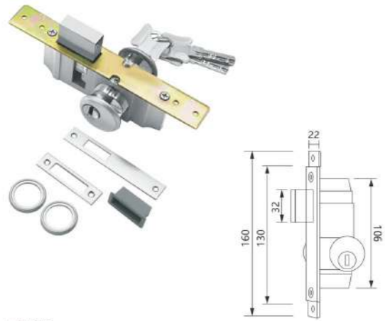
LB-15 Body Material: Aluminum alloy
