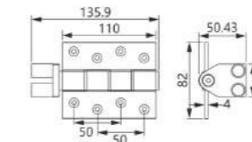
Top guide
