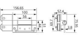
Bottom roller
