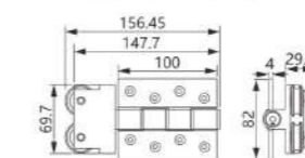
Bottom roller
