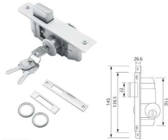
LB-15-1 Body Material: Aluminum alloy
